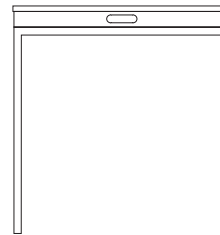
Fällbord, 1-pack Folding table, 1-pack 折りたたみ式テーブル 1 個入 w78/d96/h71 cm
